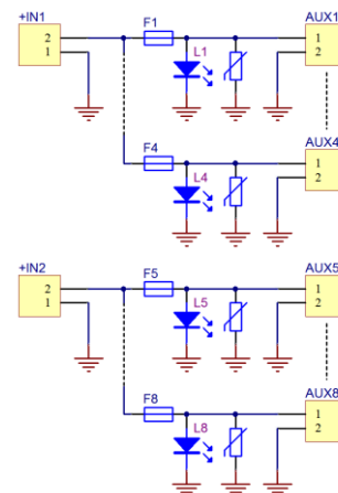
Rys.2. Schemat elektryczny.
